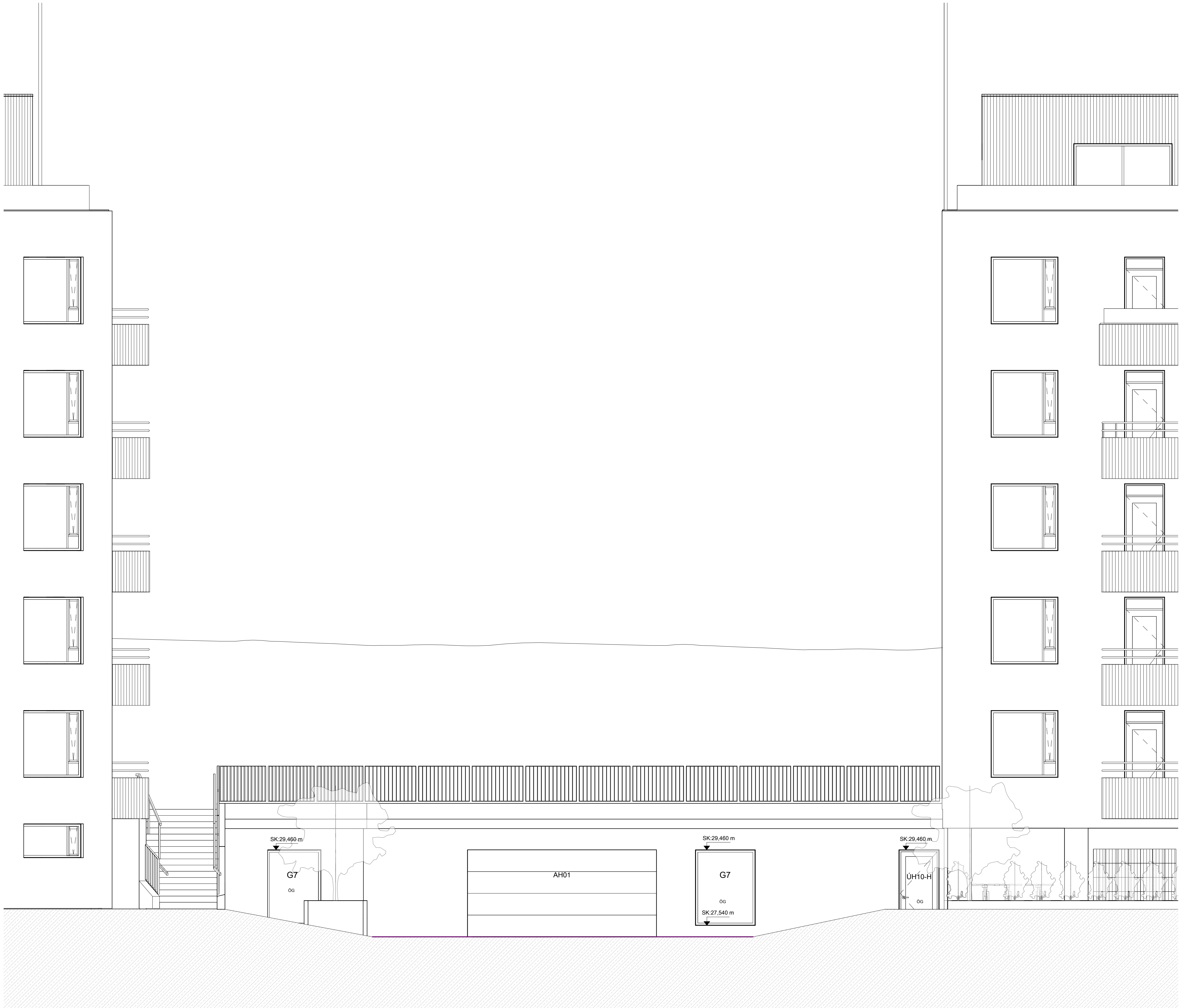
Norður. - bílakjallari mkv: 1 : 50
