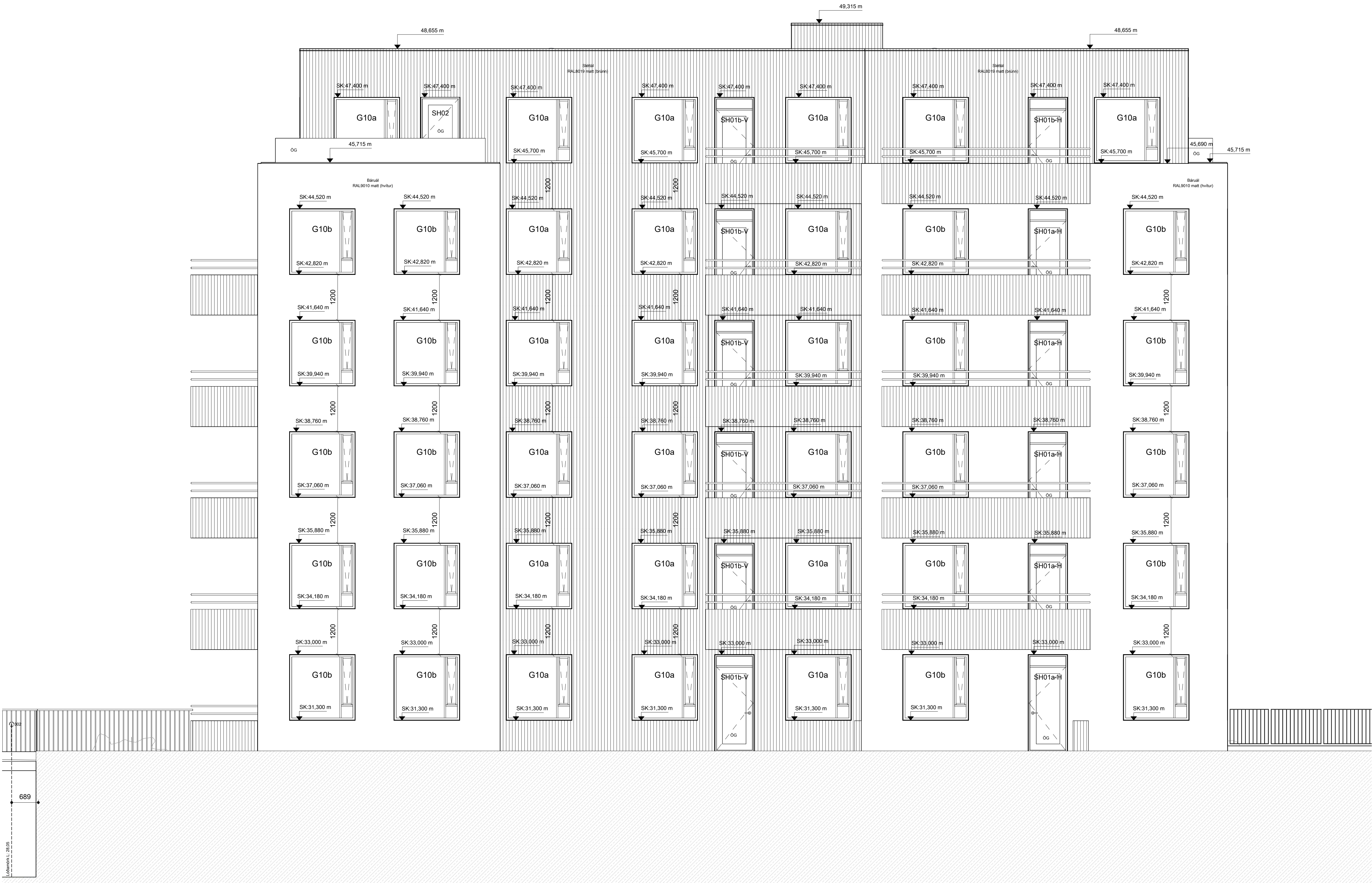
Suður. - Baughamar 7 mkv: 1 : 50
